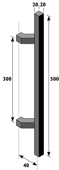
Standard Stoßgriffpaar Eckig
