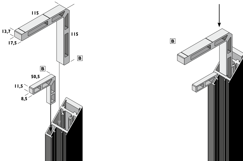
Eckverbindung Türrahmen
