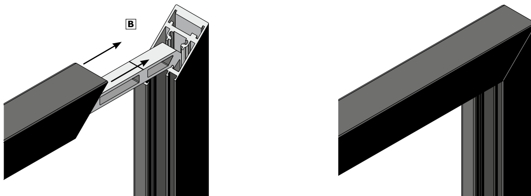
Eckverbindung Türrahmen
