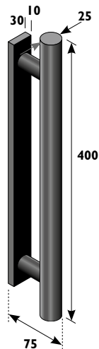
Griffstange Gerundet
